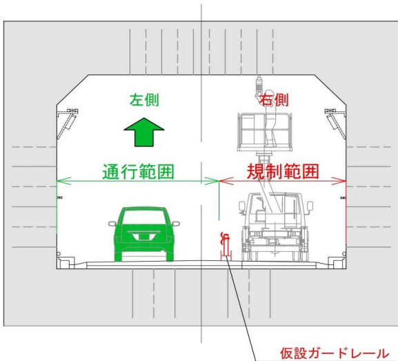
右側規制時 標準断面図 (半田行き)
