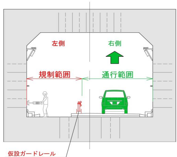
左側規制時 標準断面図 (半田行き)
